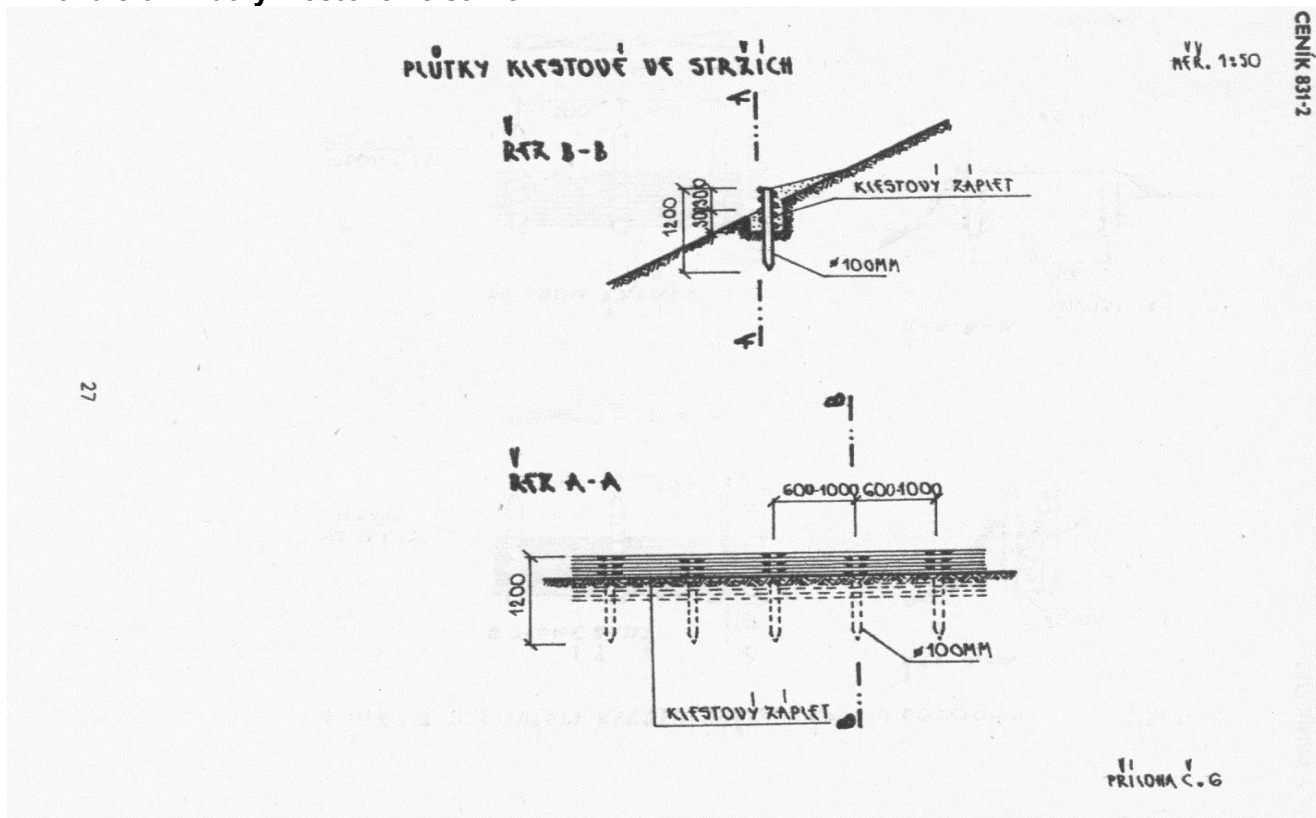
Príloha č.6 - Plůtky klestové ve stržích
