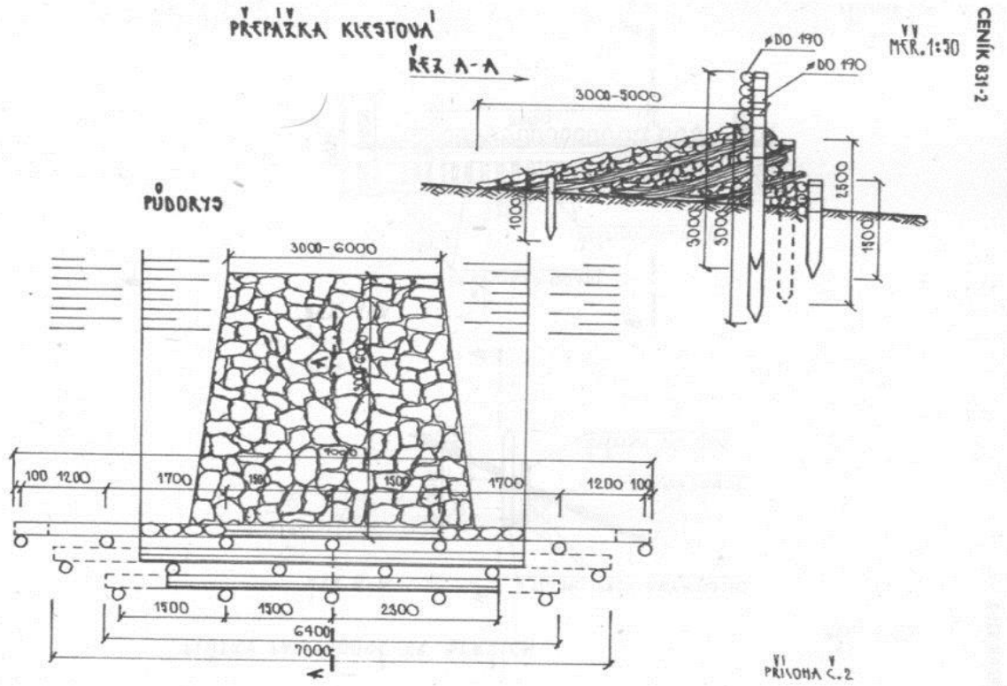
Příloha č.3 - Plůtky tyčové ve stržích
