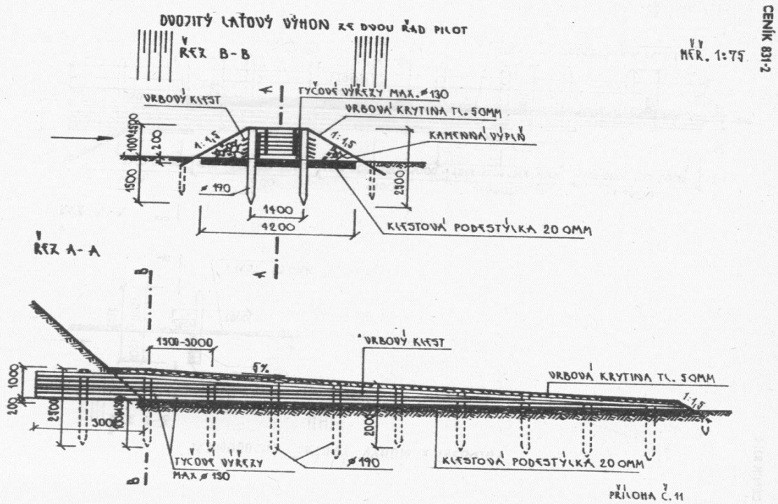
Příloha č.11 - Dvojitý laťový výhon ze dvou řad pilot
