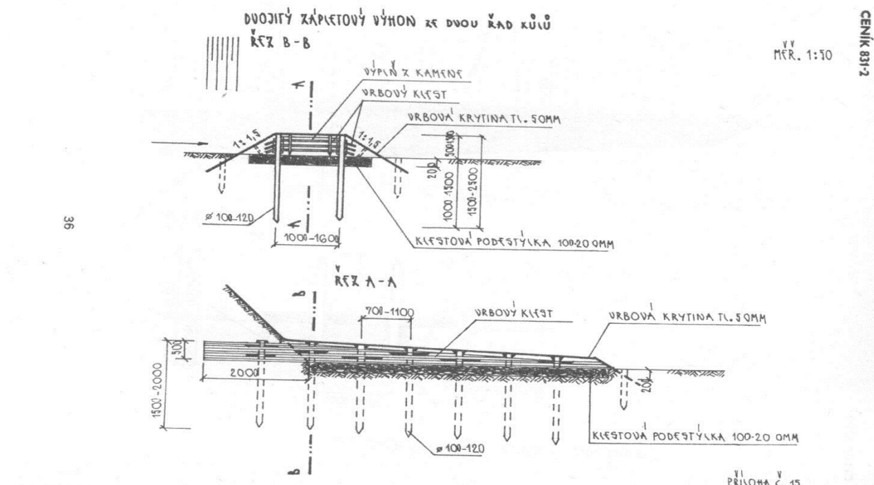
Příloha č.15 - Dvojitý zápleťový výhon ze dvou řad kůlů
