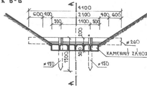
ŘEZ B-B
