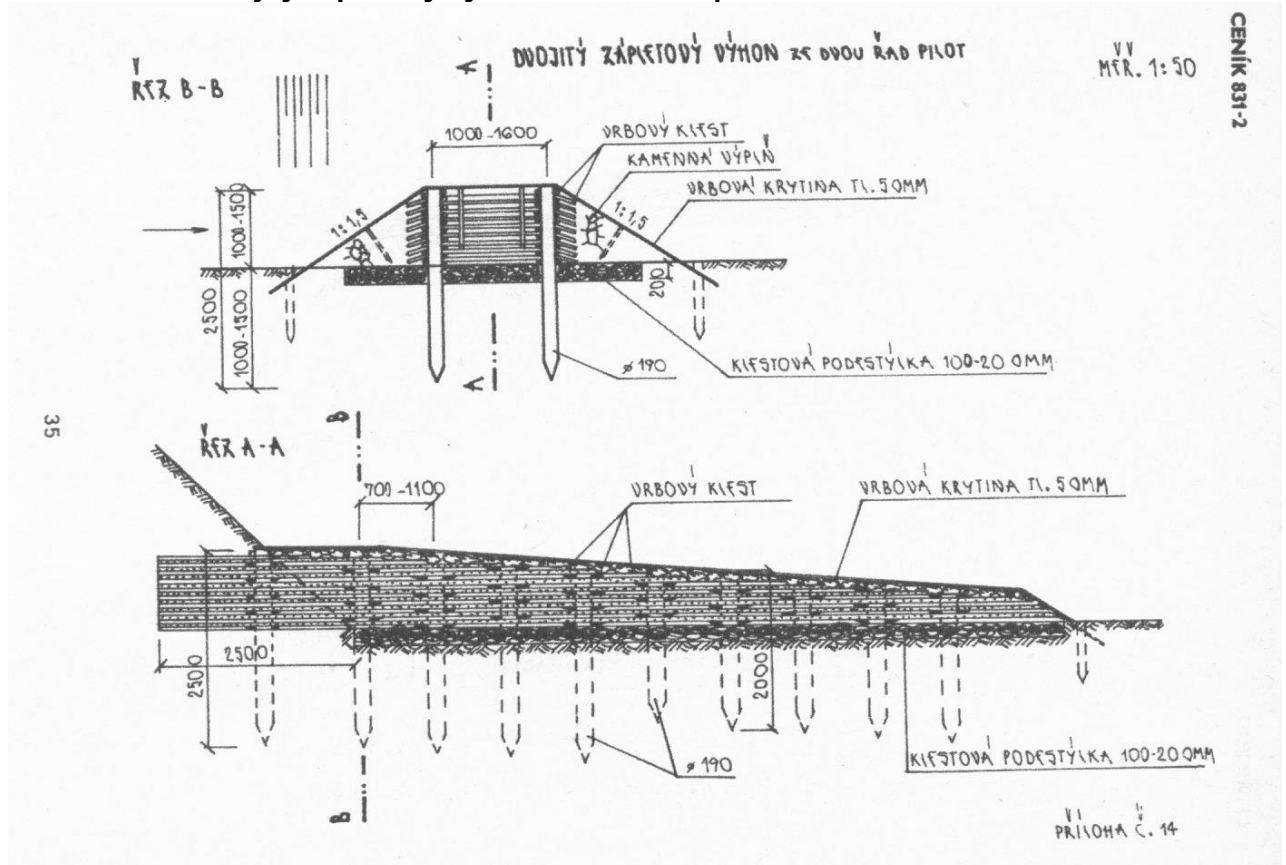
Příloha č.14 - Dvojitý zápleťový výhon ze dvou řad pilot
