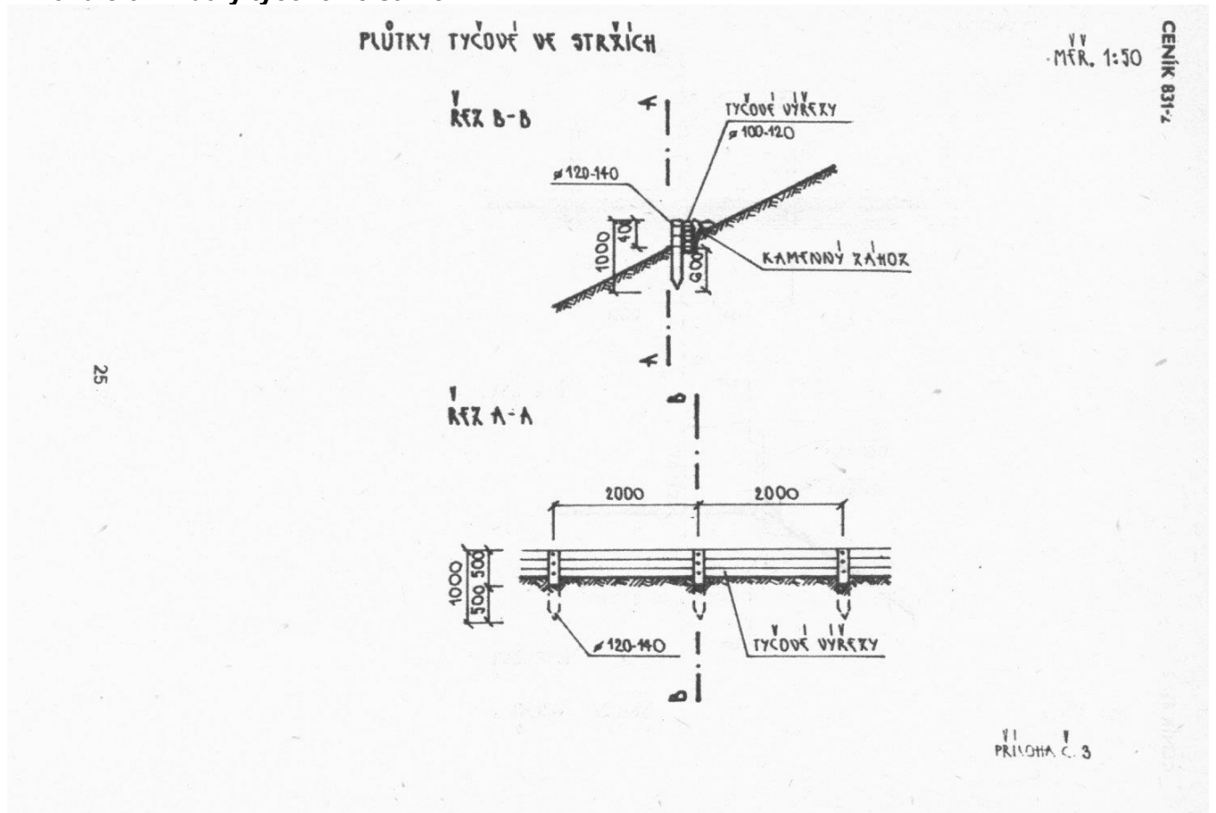
Příloha č.3 - Plůtky tyčové ve stržích
